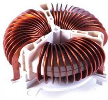
三相共模电感
